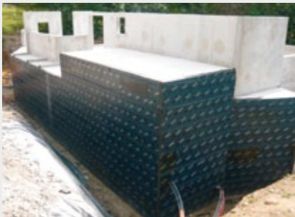
Pose des panneaux Board avec la colle PC® 56
