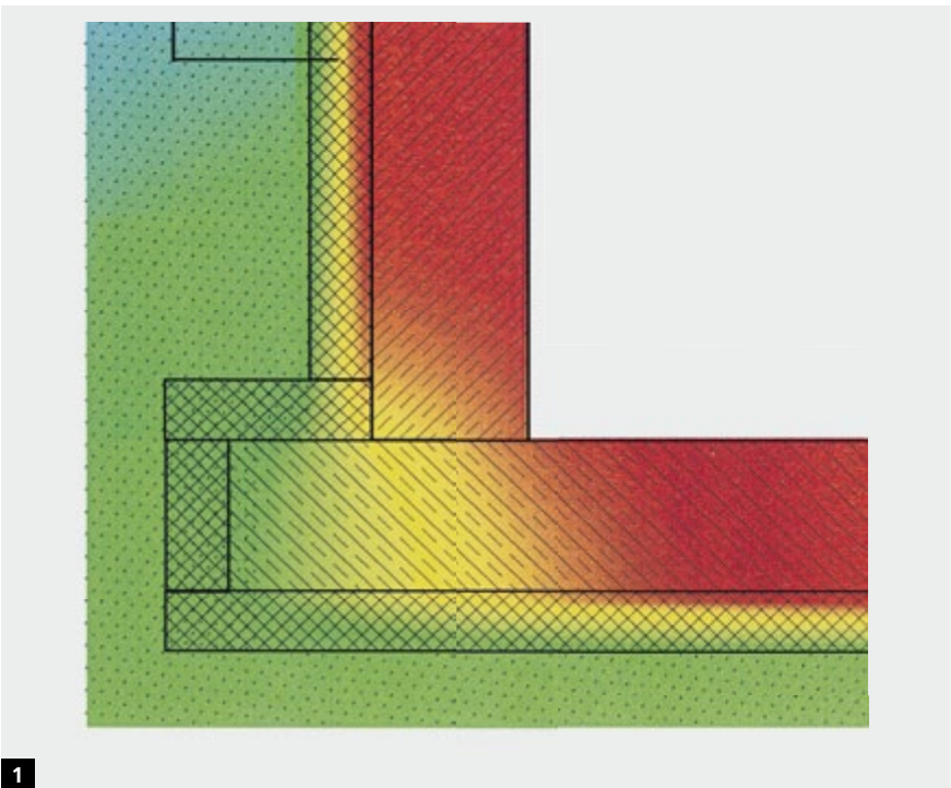
1 Fondations: thermographie avec isolation FOAMGLAS®
